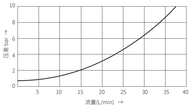
\Delta p - q_v 特性曲线 (A1 到 A2)
