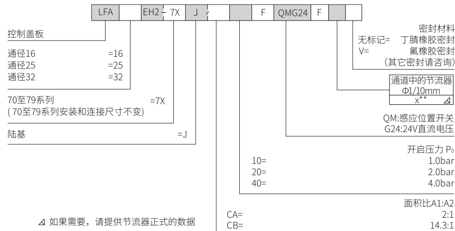
LFA...EH2... 规格 16至32
