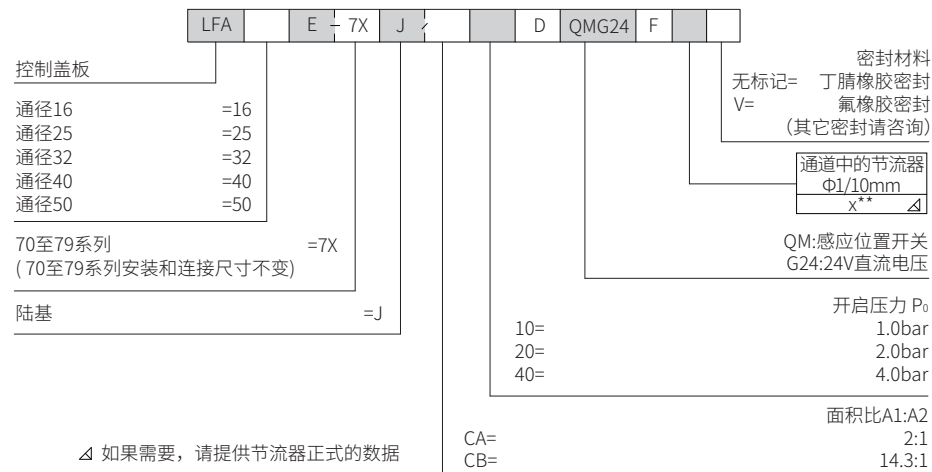
LFA...E... 规格 16至50
