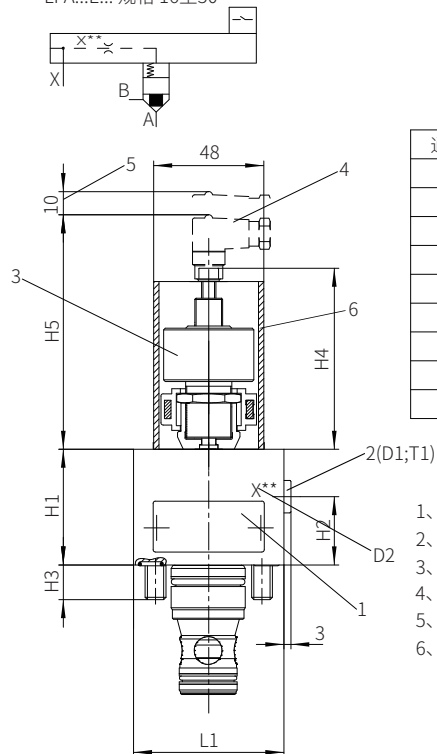
LFA...E... 规格 16至50
