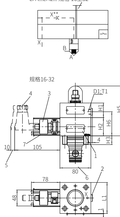
LFA...EH2... 规格 16至32
